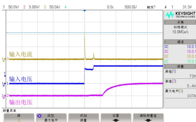
图 1.未使用限流电阻 R3 上电瞬间输入、输出波形 输入电流峰值 107A
