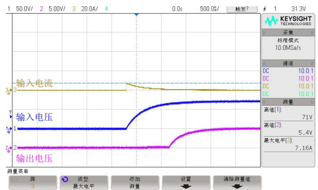
图 2.使用限流电阻 R3 后上电瞬间输入、输出波形 输入电流峰值降至 7.16A
