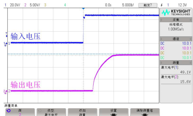
图 6. VIN=48V，VOUT=15V/0.2A
