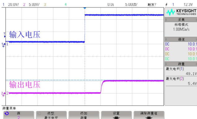
图 5. VIN=48V，VOUT=5V/0.3A
